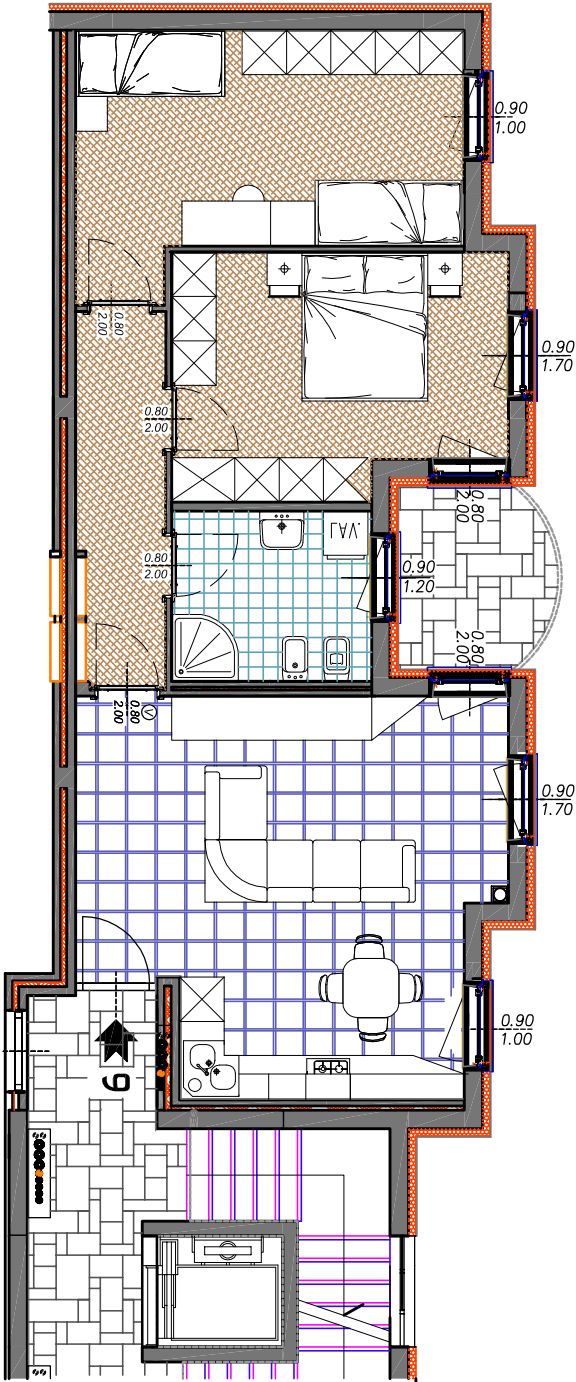
PIANTA PIANO SECONDO SOPPALCO
